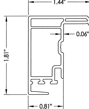
7 LOCK STILE
